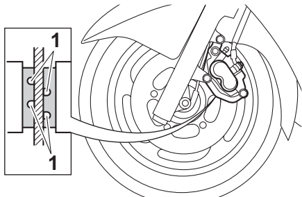
1. Индикатор износа
